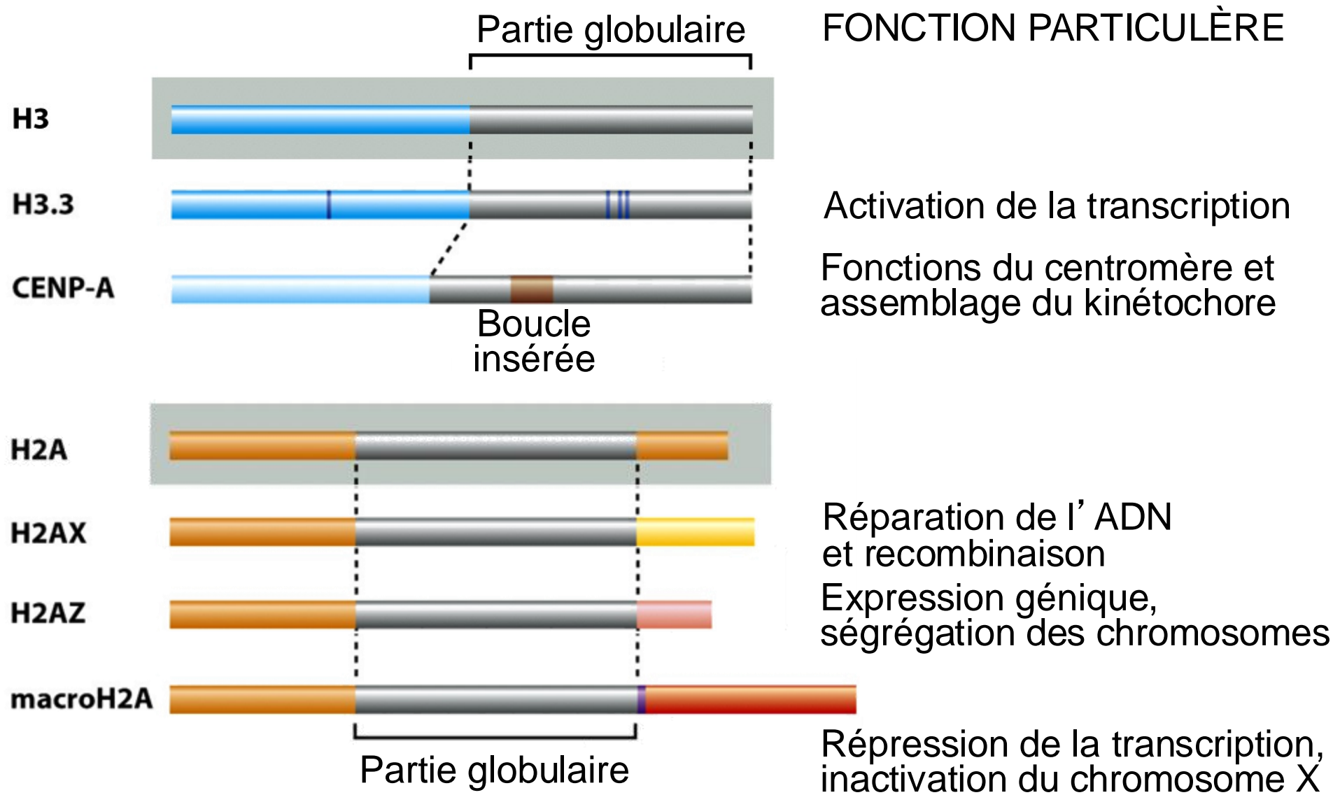
Structure et fonction de quelques variants d'histones comparée à celle des histones qu'ils remplacent
