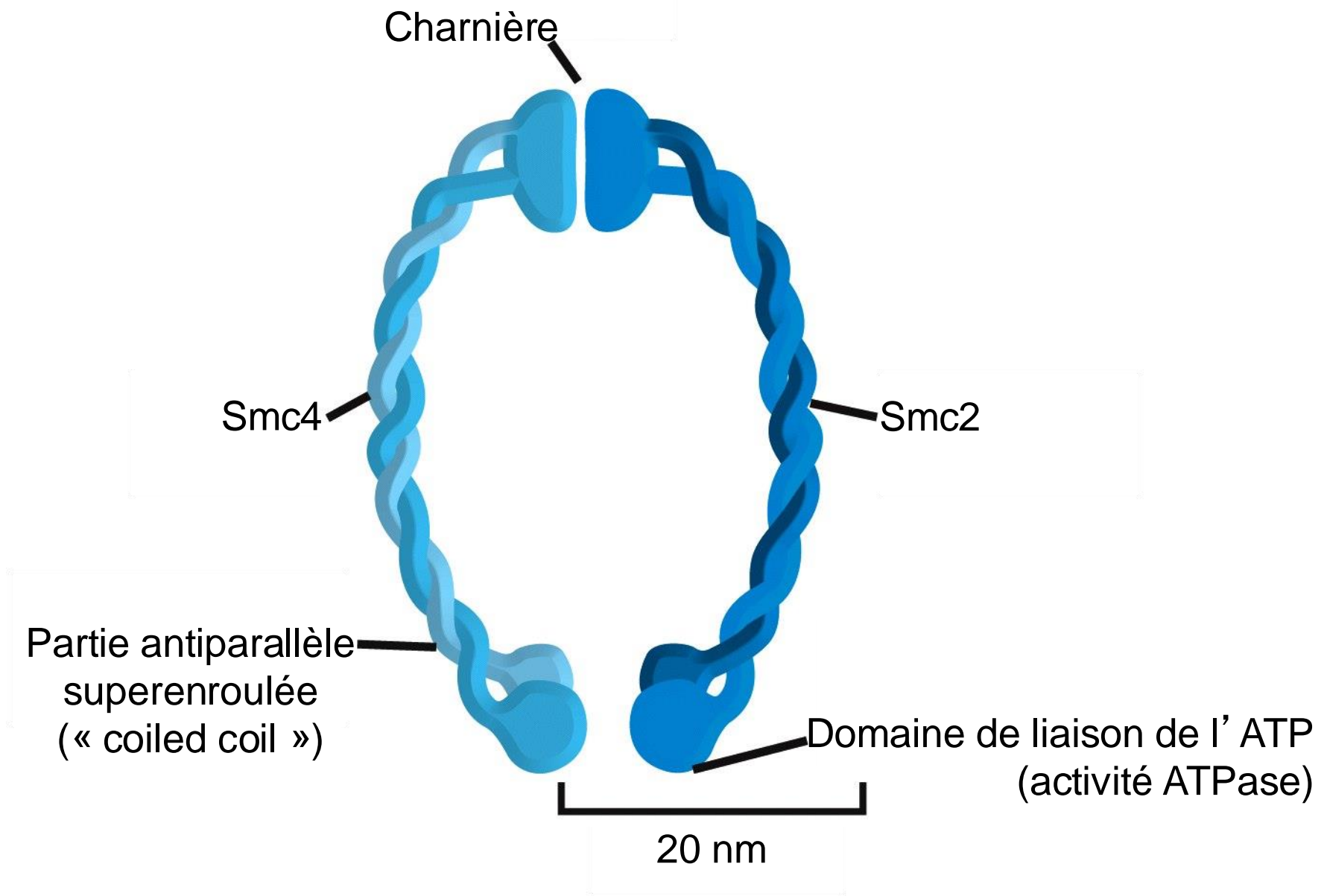
Structure du dimère de SMC
